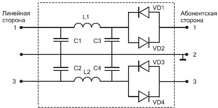
Рис. 16.7. Схема защиты № 1 (C1-C4 — 0,022 пФ; L1, L2 — 1,5 мкГн; VD1-VД4 — КД 102А)
