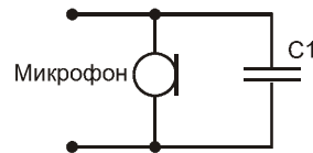
Рис. 16.12. Схема защиты № 6 ( C_1 — 0,01–0,05 пФ)
