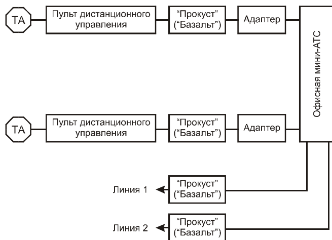
Рис. 16.6. Схема включения постановщика помех в офисную телефонную сеть
