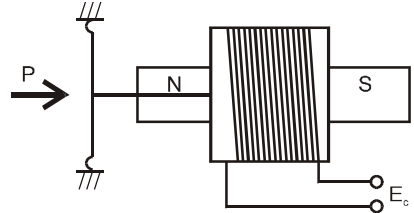
Рис. 6.16. Возникновение ЭДС в электродинамическом микрофоне
