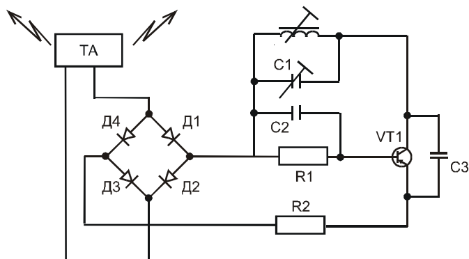
Рис. 12.7. Схема радиозакладки с однотранзисторным генератором несущей частоты
