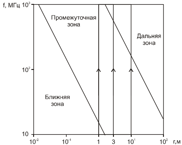
Рис. 11.7. Зависимость расстояний до границ зон от частоты ПЭМИ при x = 3
