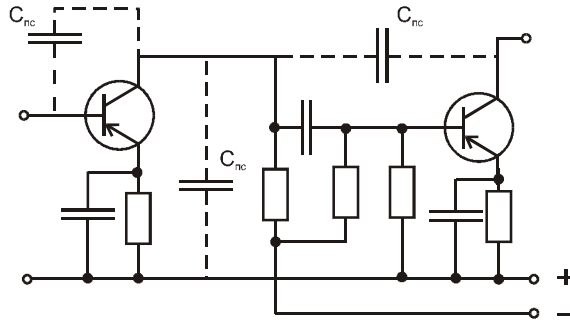
Рис. 7.1. Схема возникновения паразитной емкостной связи
