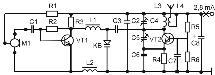
Рис. 12.2. Принципиальная схема типичной радиозакладки
