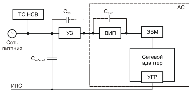
Рис. 14.2. Схема образования каналов проникновения НСВ
