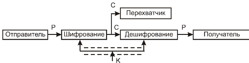
Рис. 18.3. Поток информации в криптографической системе, обеспечивающей секретность
