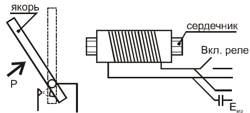
Рис. 6.18. Схема возникновения ЭДС на реле
