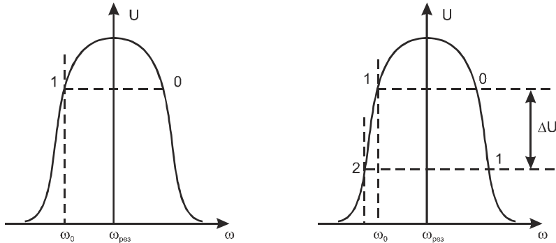
Рис. 6.10. Амплитудно-частотная характеристика при использовании резонансной схемы
