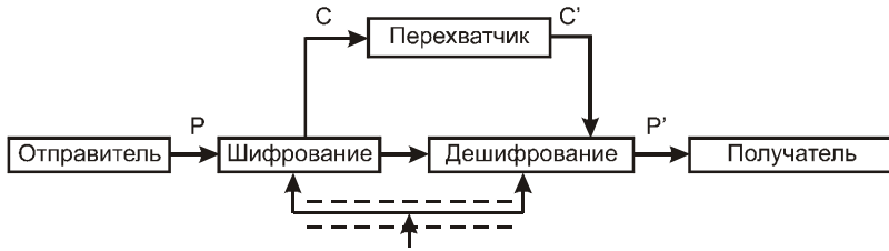
Рис. 18.4. Поток информации в криптографической системе, обеспечивающей имитостойкость
