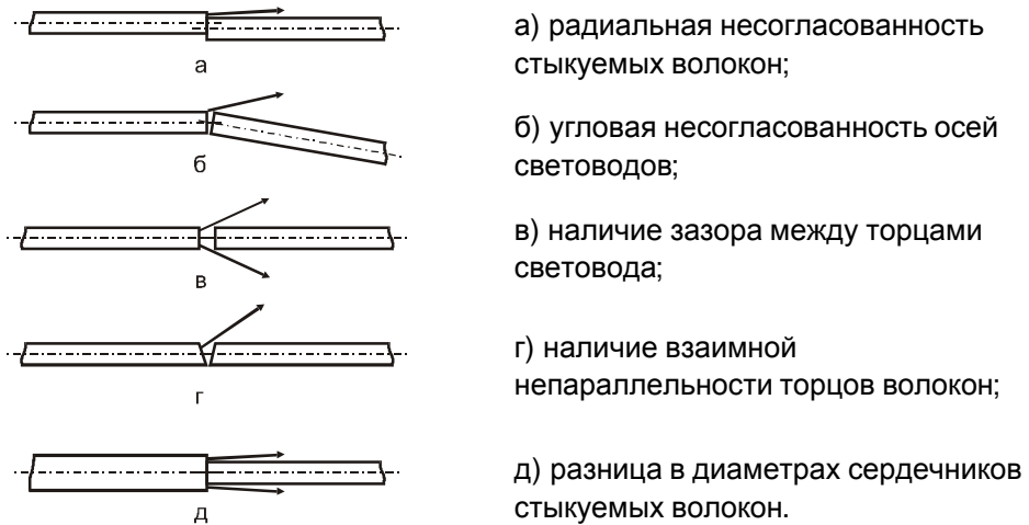
Рис. 4.7. Причины возникновения излучения в ВОЛС
