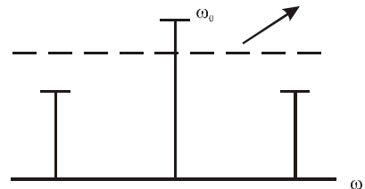
Рис. 6.8. Излучение модулированного сигнала
