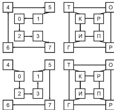
Рис. 18.5. Схема шифрования перестановкой по маршрутам Гамильтона.
