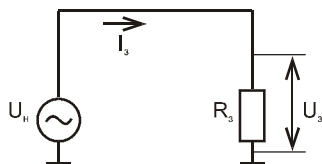
Рис. 7.4. Схема заземления
