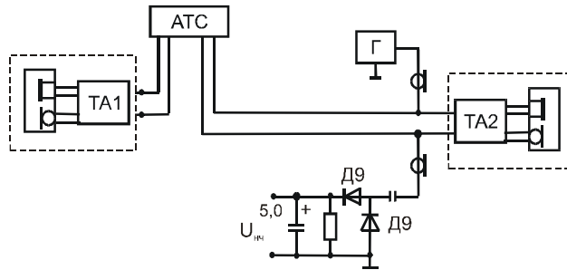
Рис. 12.5. ВЧ навязывание при положенной трубке
