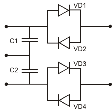
Рис. 16.10. Схема защиты № 4 ( C_1, C_2 — 0,02; VD1–VD4 — КД 102А)
