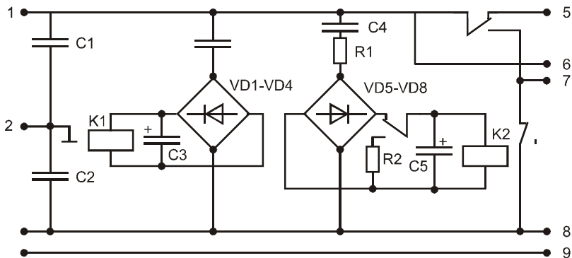
Рис. 16.8. Схема защиты № 2 (C1, C2 — 0,22 пФ; C4 — 5,0 пФ; C5 — 20...50 пФ; R1 — 2,4 кОм; R2 — 100 Ом; VD1-VД8 — КЦ 405Д; K1 — РЭС15 РС4.591.001; K2 — РЭС9 РС4.524.205172)
