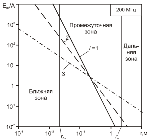
Рис. 11.6. Напряженность электрического поля на частоте 200 МГц
