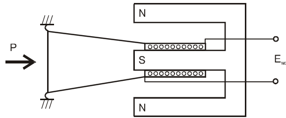
Рис. 6.19. Схема возникновения ЭДС на громкоговорителе
