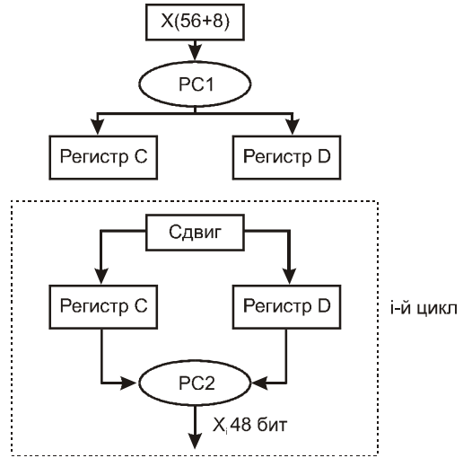
Рис. 18.8. Формирование подключей
